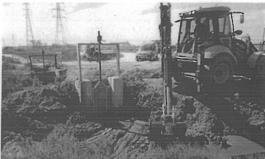
Installation d'une martelière pour faciliter la gestion hydraulique
